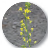
BBCH 65
