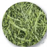
BBCH 79
